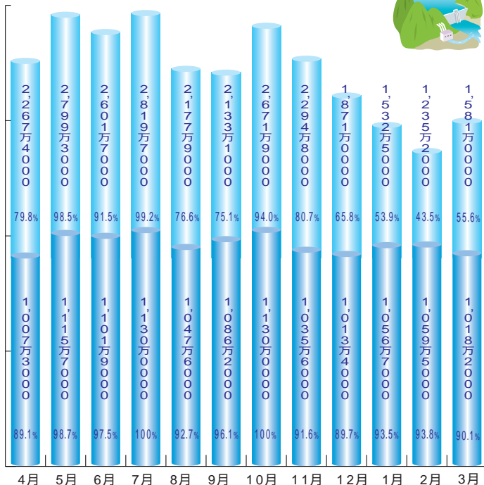
平成18年度 ダム水源状況（月平均）
